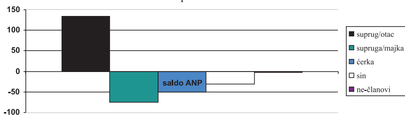
Grafikon br. 6: Saldo učešća u ANP u porodici
