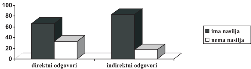
Grafikon br. 2: POREĐENJE DIREKTNIH I INDIREKTNIH ODGOVORA Poređenje direktnih i indirektnih odgovora
