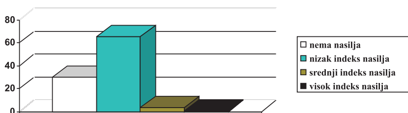
Grafikon br. 4: Učestalost ASIN u uzorku
