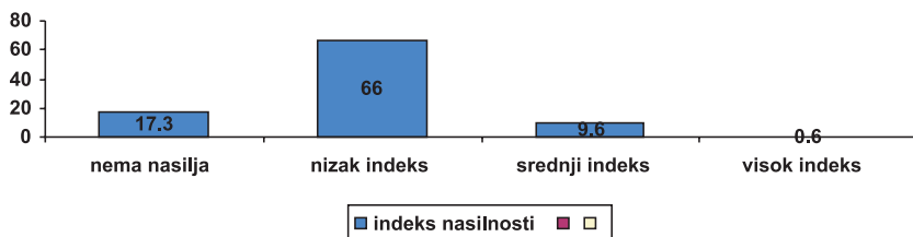
Grafikon br.5: Korigovani rezultati u učestalosti ASIN
